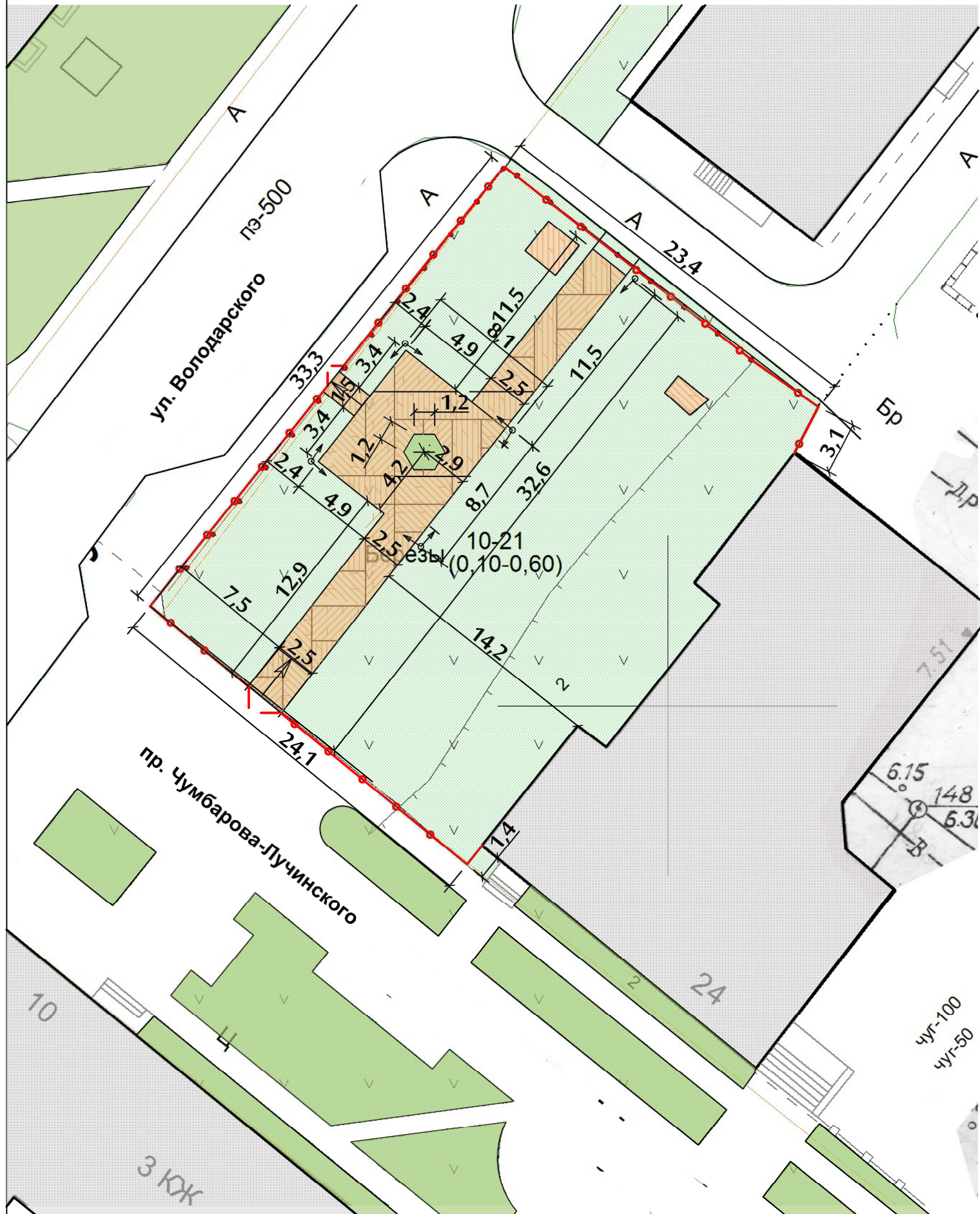
Разбивочный план дорожек:
